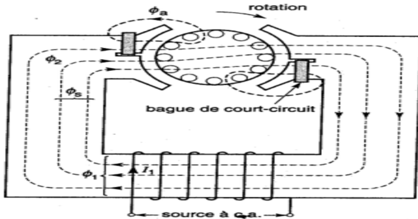
Figure 17 Construction d'un moteur à bagues de court-circuit.
