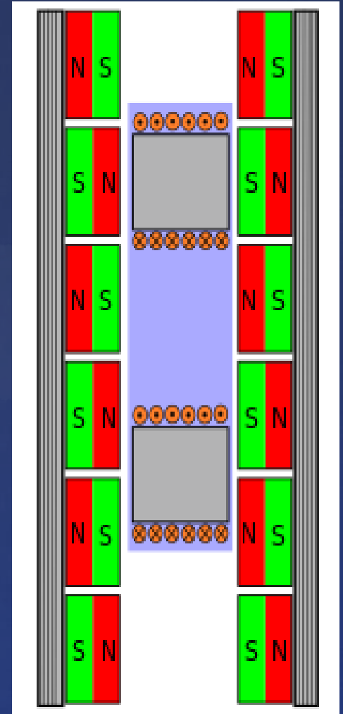
Moteur linéaire synchrone alimenté en courant alternatif en quadrature
