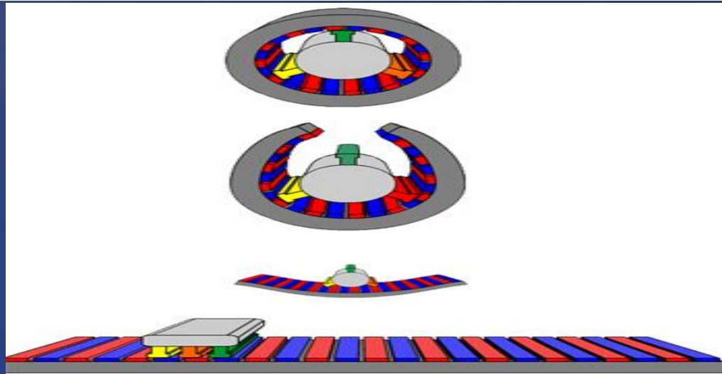
Mise à plat d'un moteur rotatif synchrone triphasé
