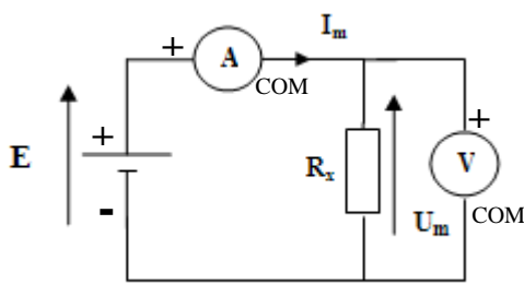
Montage Aval (courte dérivation)
