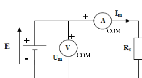
Montage Amont (longue dérivation)
