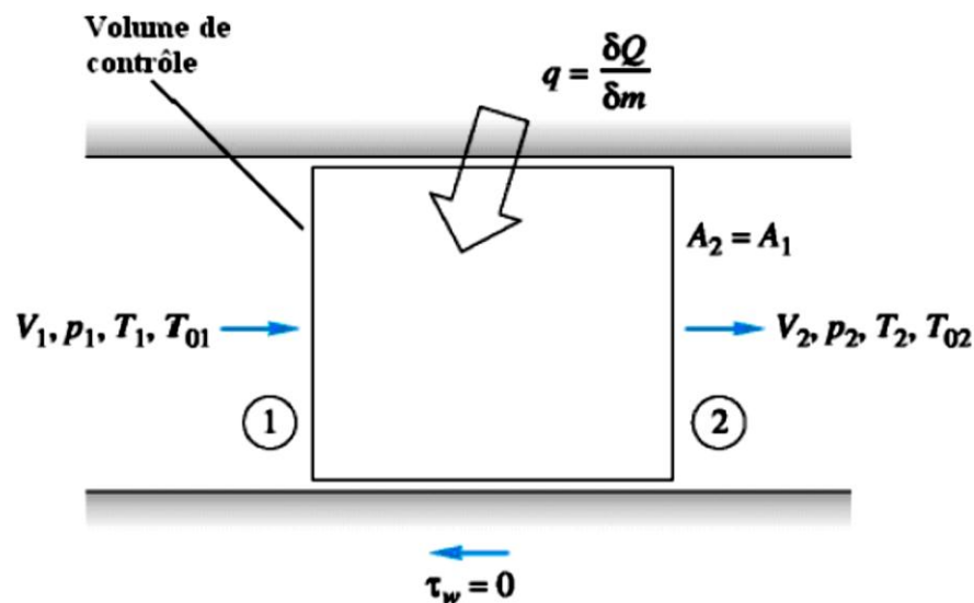
Fig. 6-1 : Volume de contrôle élémentaire pour un écoulement sans friction dans une conduite de section constante avec transfert de chaleur.
