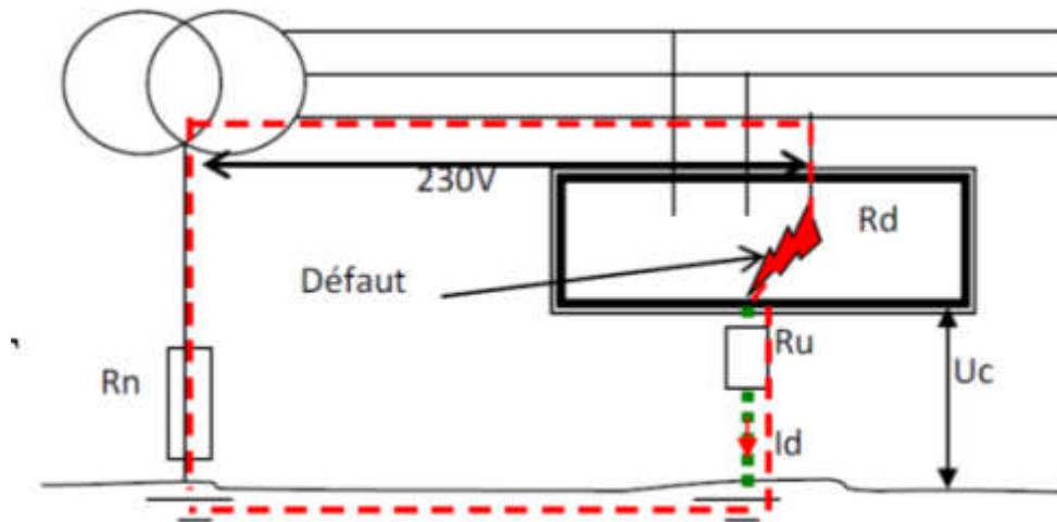
Régime TT
