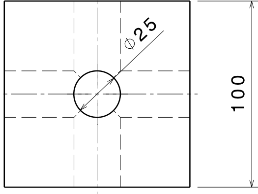
Vue de gauche Echelle : 1:2
