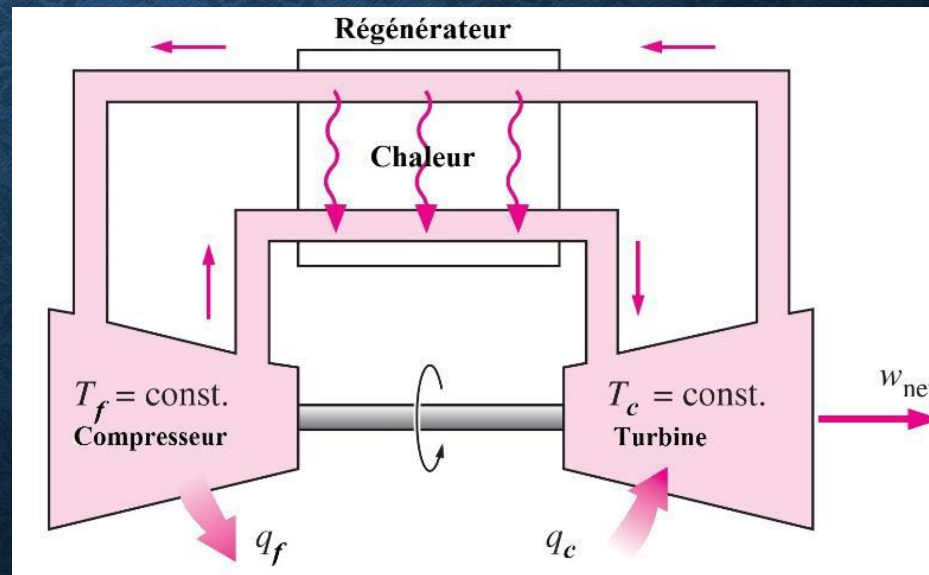
Moteur fonctionnant avec le cycle d’Ericsson.
