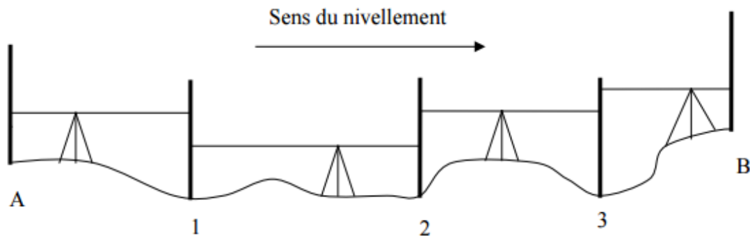
Figure 3 – Nivellement par cheminement.
