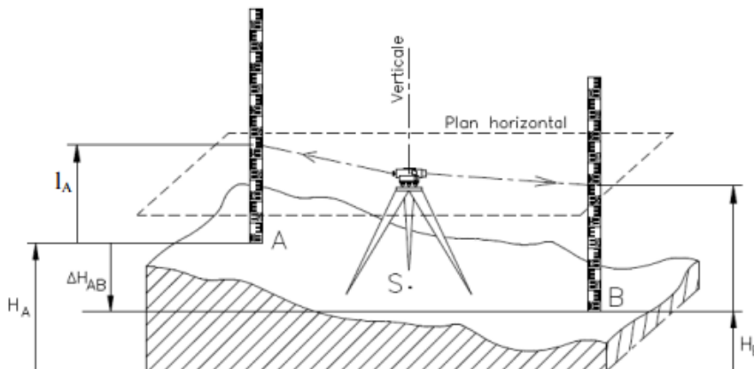
Figure 2 – Principe de base de nivellement direct
