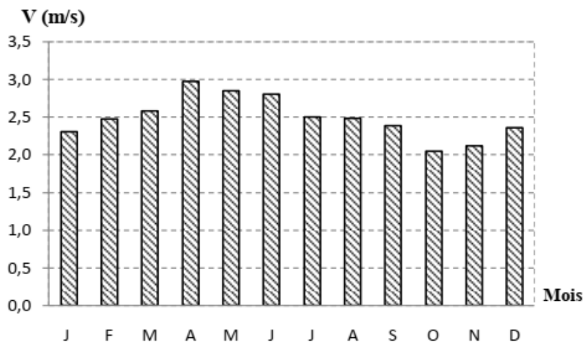
Figure 12 : Moyenne mensuelle des vitesses du vent moyen de la station X
